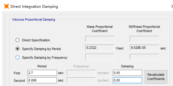
图 8 有桥墩模型调整后的瑞利阻尼
