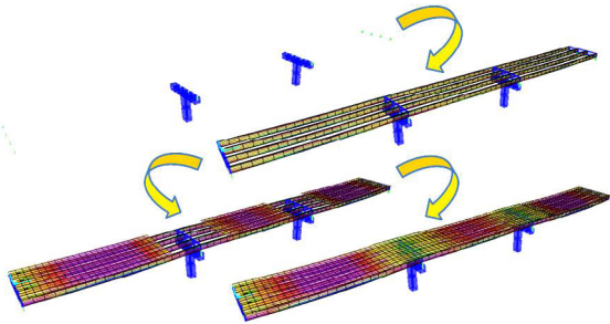
图 1.2-2 CSiBridge
